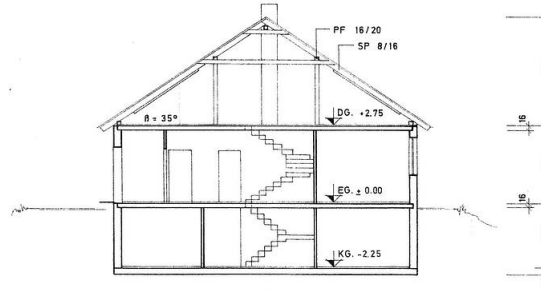
SCHNITT WOHNHAUS
